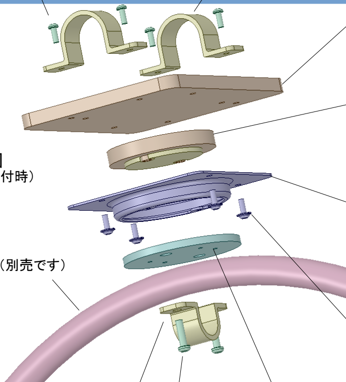
⑦ アンテナ取付丸板 [1個]
